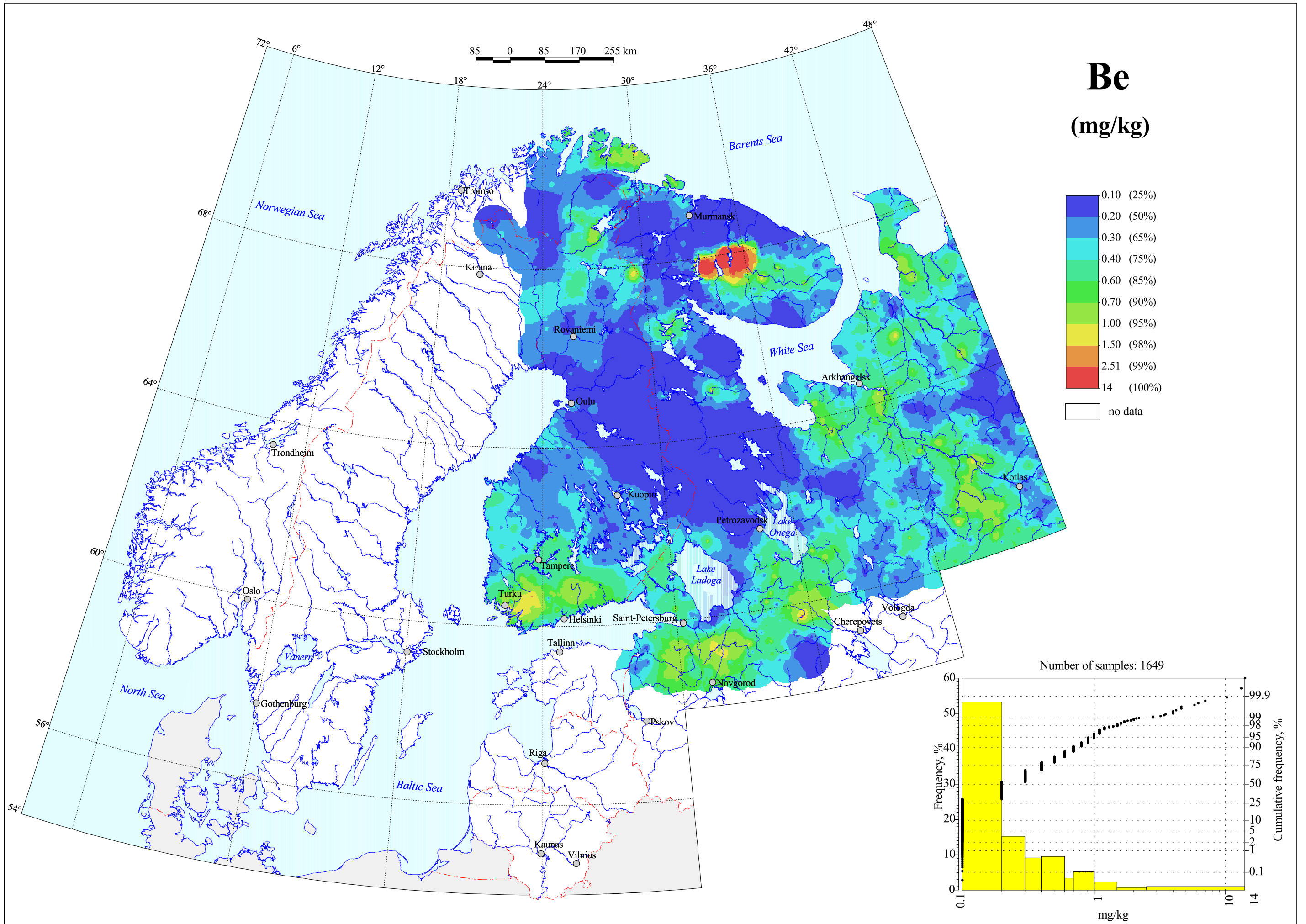
Beryllium in C-horizon, Grain Size <2 mm, Aqua regia Extraction
